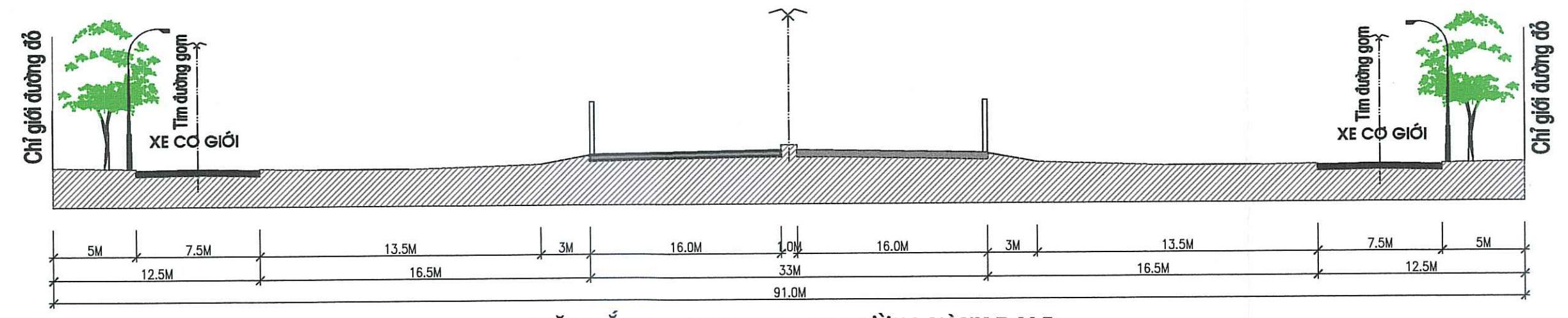
MẶT CẮT A - A QUY HOẠCH ĐƯỜNG VÀNH ĐAI 5
